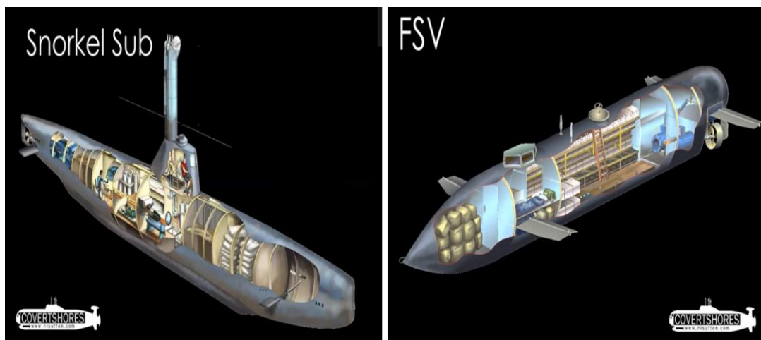
Figura 10. Sumergibles para tráfico de CHC. Fuente: Sutton H. (2022)
